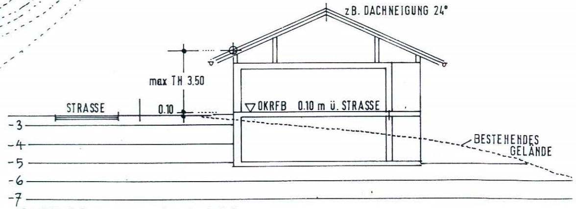
QUERSCHNITT M 1:200 FÜR GEBÄUDE AUF FL.NR. 5664
